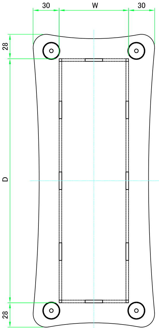
上カバー / Top cover
