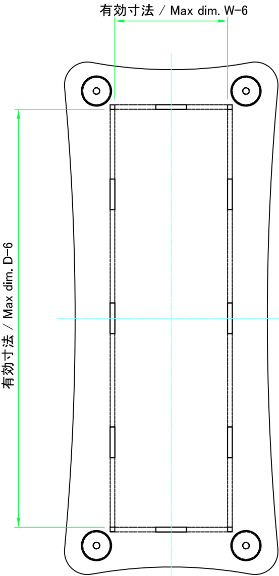
下カバー / Bottom cover
